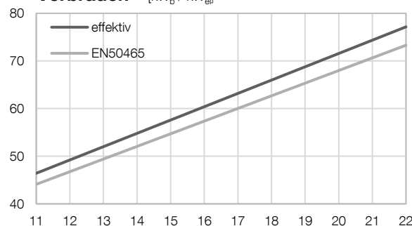
Verbrauch 3) [kW b / kW el ]
