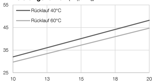
Verbrauchsskurven 3) [kW b / kW e ]
