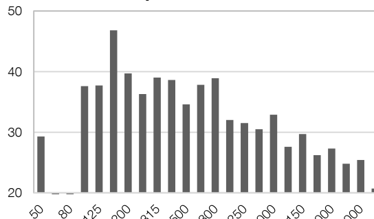
Schalldruckspektrm 6) [dB(A) / Hz]
