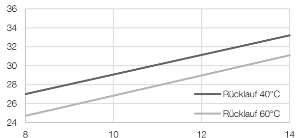
Leistungskurven [kW b / kW e ]
